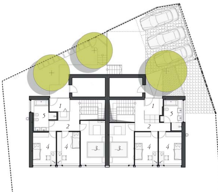
Pôdorys 1. np – prízemie
