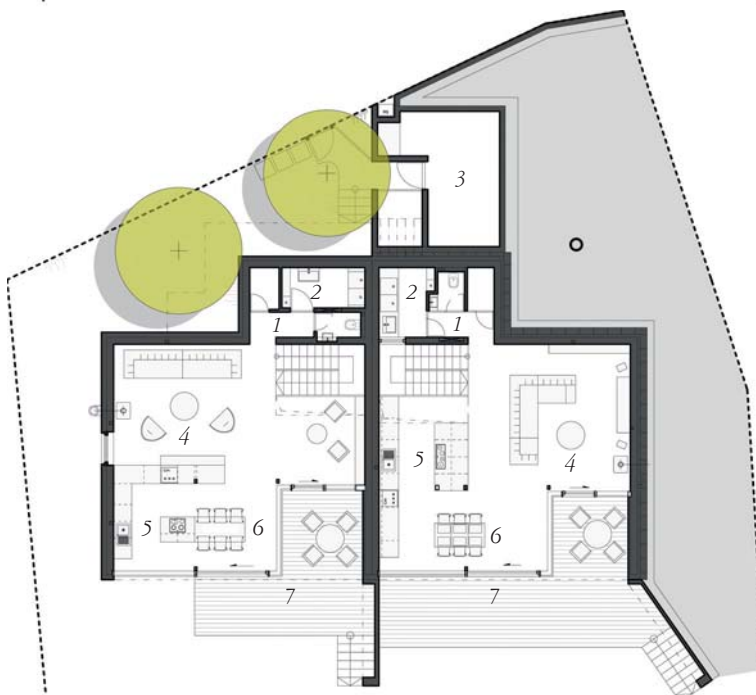
Pôdorys 1. pp – čiastočne zapustené podlažie
