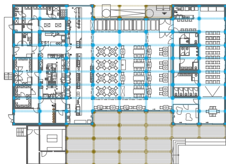
Pôdorys 1. np
